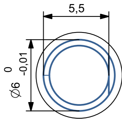
D 字型轴尺寸 比例 5 : 1
